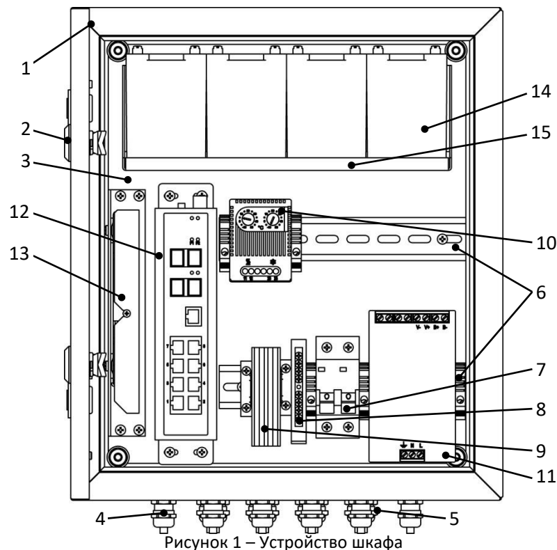
Рисунок 1 – Устройство шкафа
