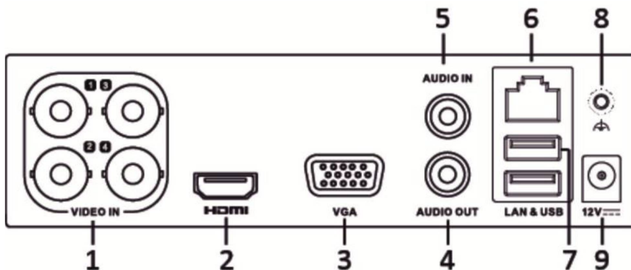
Рис 1.2 Задняя панель
