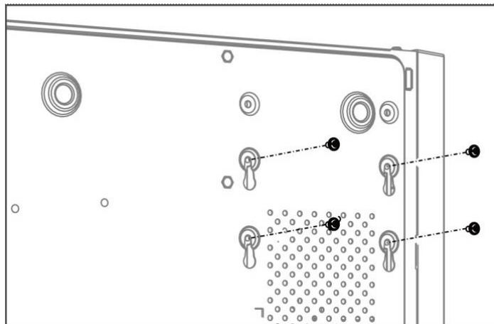
Рис. 2.3 Фиксация HDD
