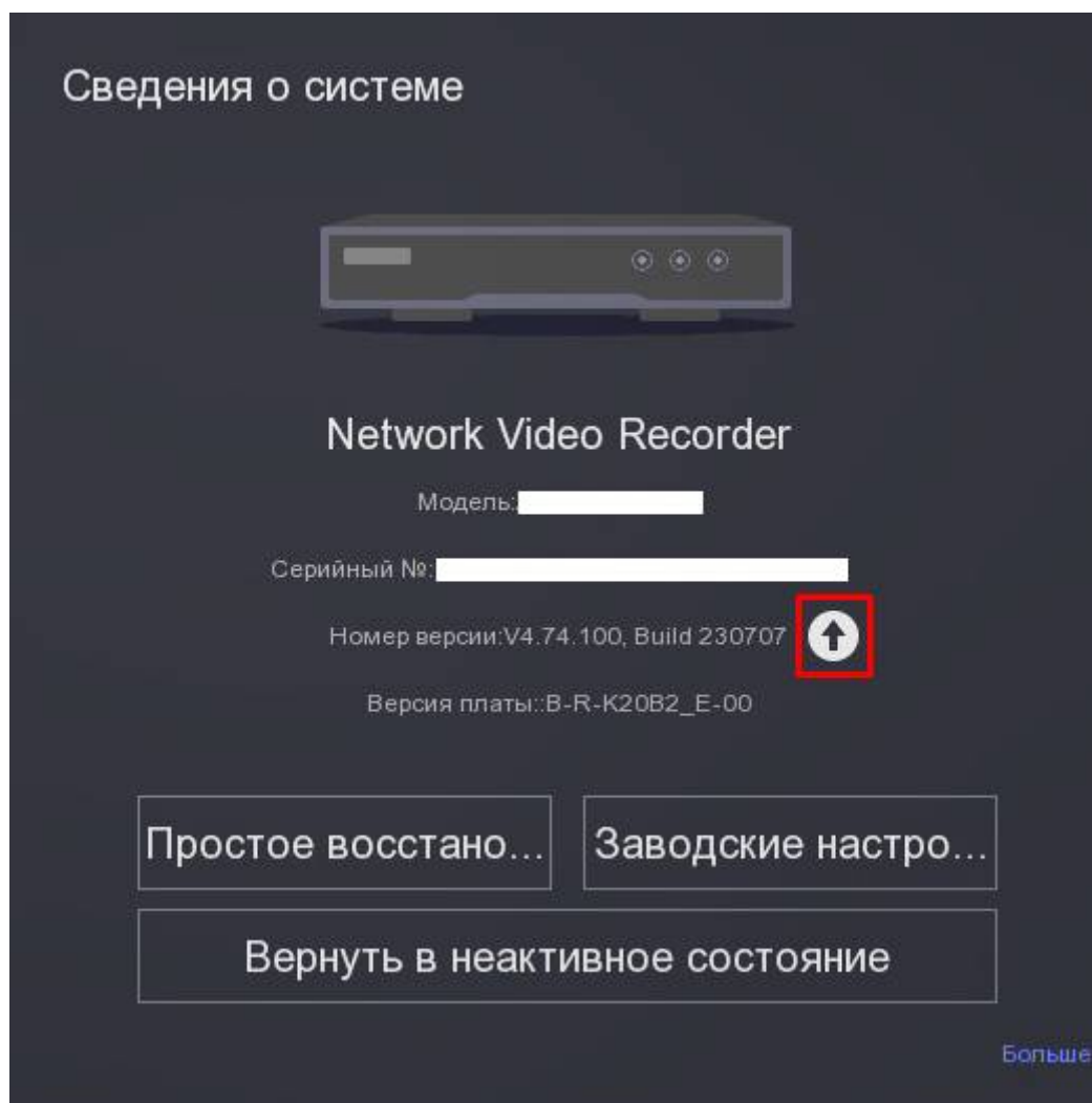
Рис. 3.37 Обновление устройства
