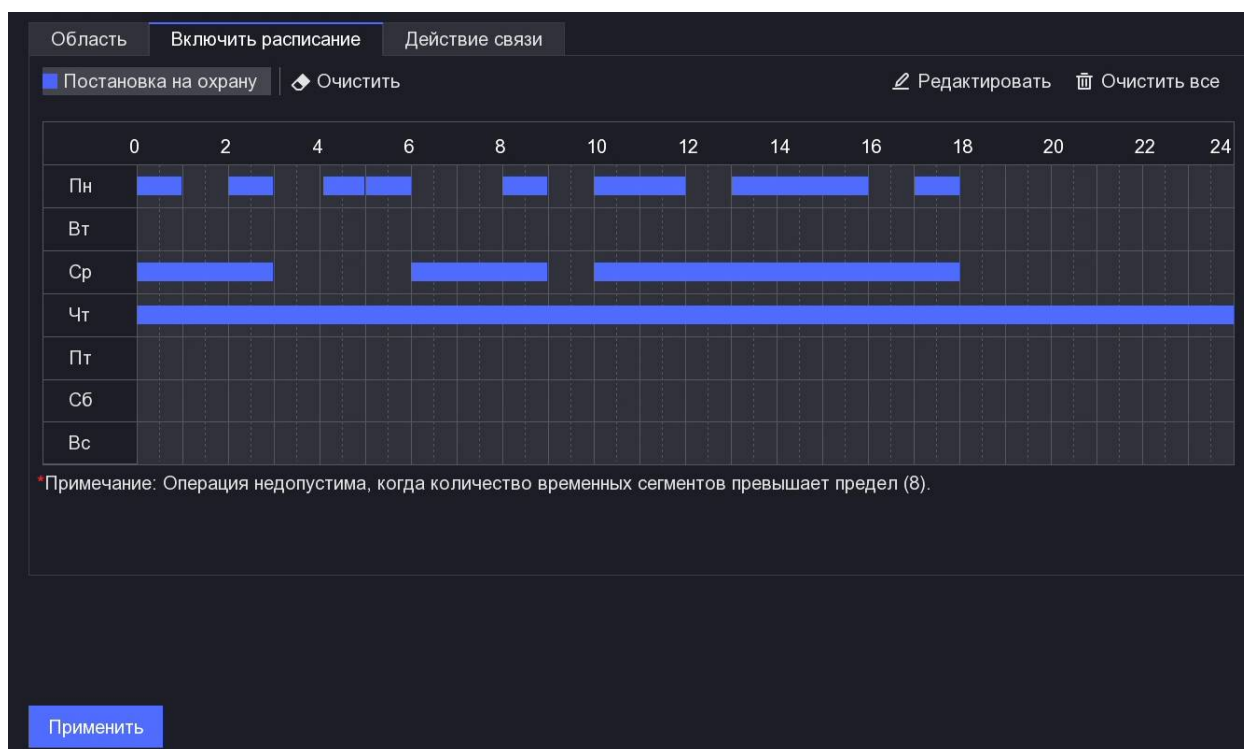
Рис. 3.25 Расписание
